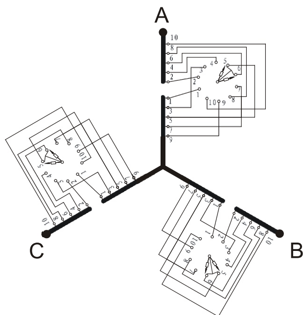
Phần dây sơ cấp và bộ chuyển mạch tự động có tải
